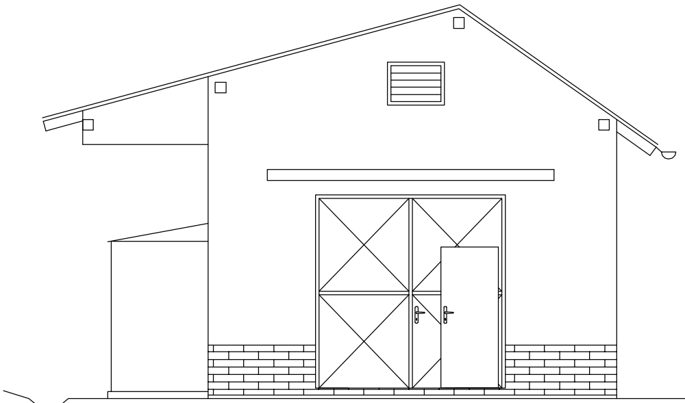
POHLED ZÁPADNÍ
